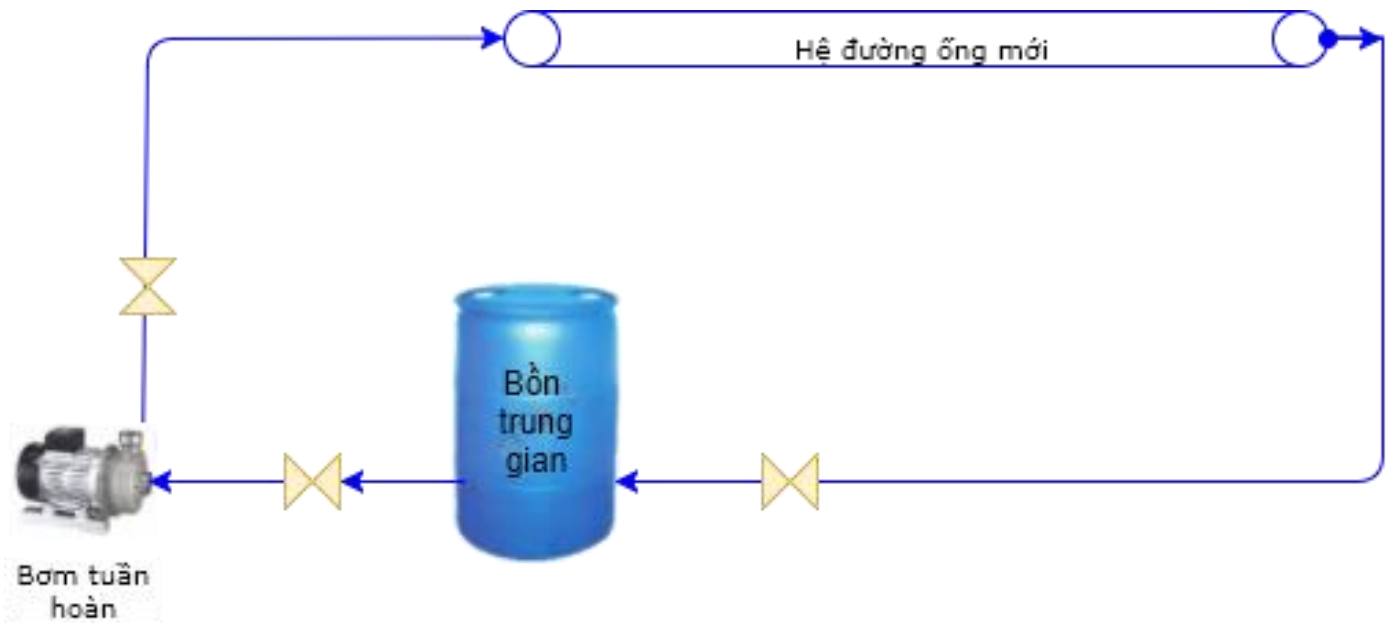
Hình 1. Sơ đồ tẩy hệ thống đường ống mới
