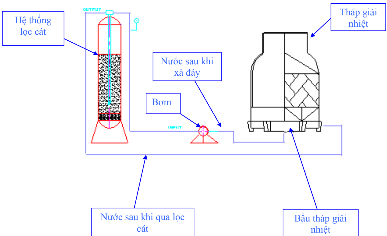
Hình 1: Sơ đồ nguyên lý của hệ thống lọc cát
