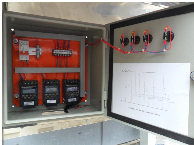
Hình 2 – Tủ điện điều khiển hệ thống châm hóa chất.
